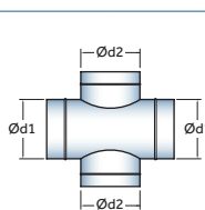
Cruz a 90°
