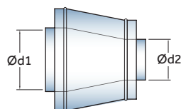
Reducción
